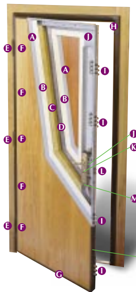
Ejemplo de una puerta acorazada certificada a2p BP 3 / Nivel 5 (según NF P 20.320)
